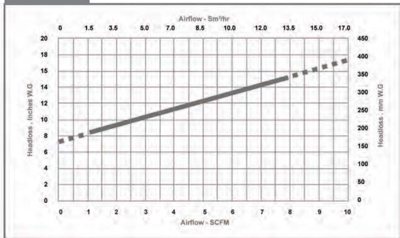
HEADLOSS PER METER
