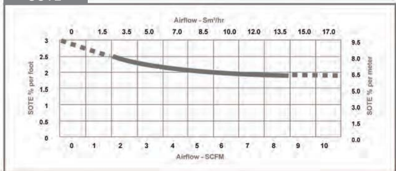
SOTE PER METER
