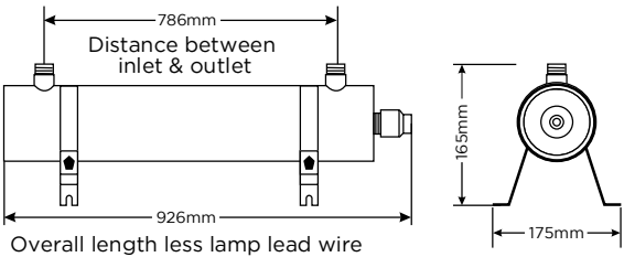
Solclear 150
