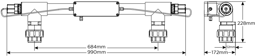
Solclear 300 V
