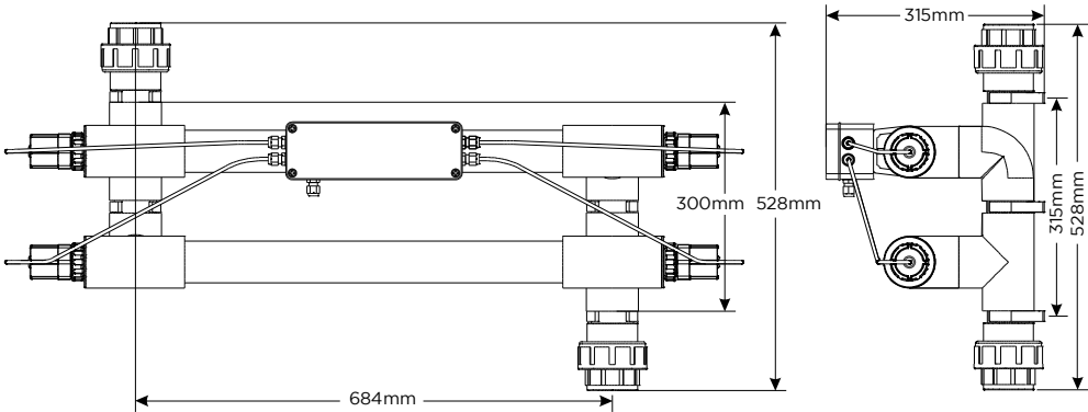
Solclear 400 V
